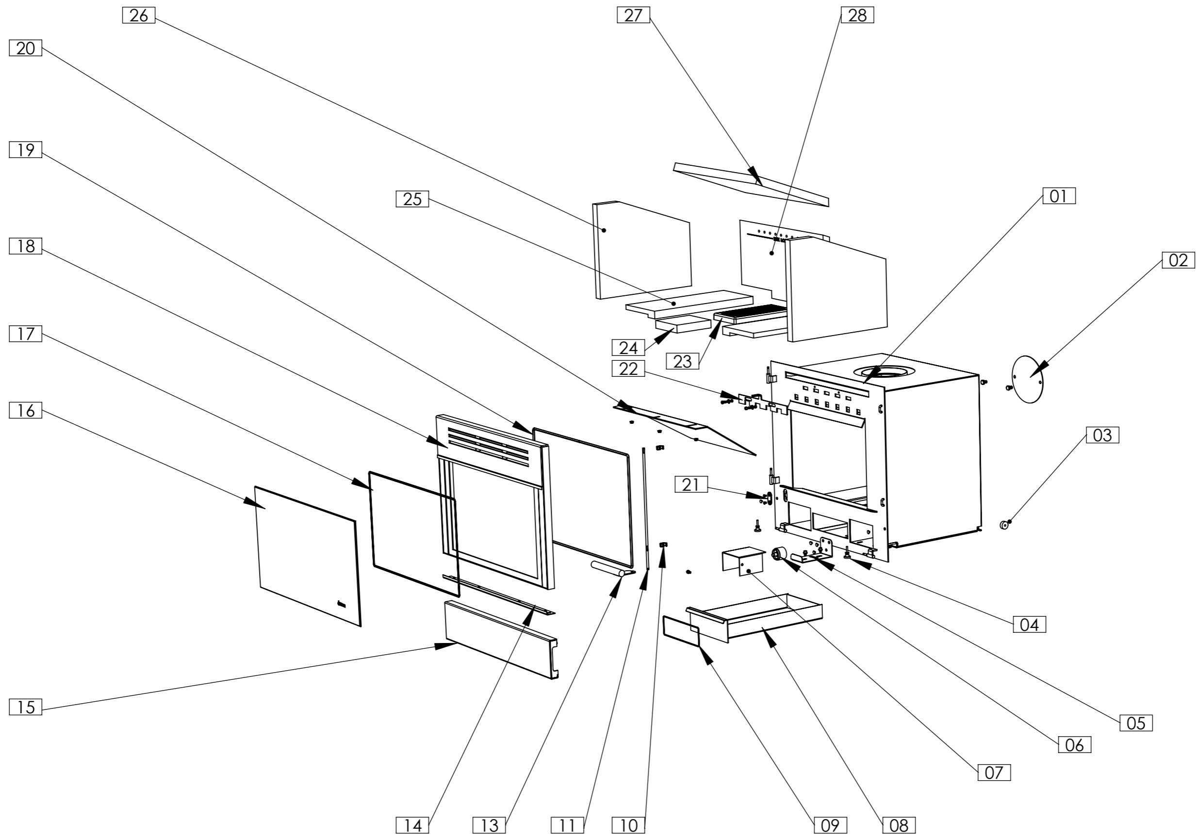
Aduro 5 explode
